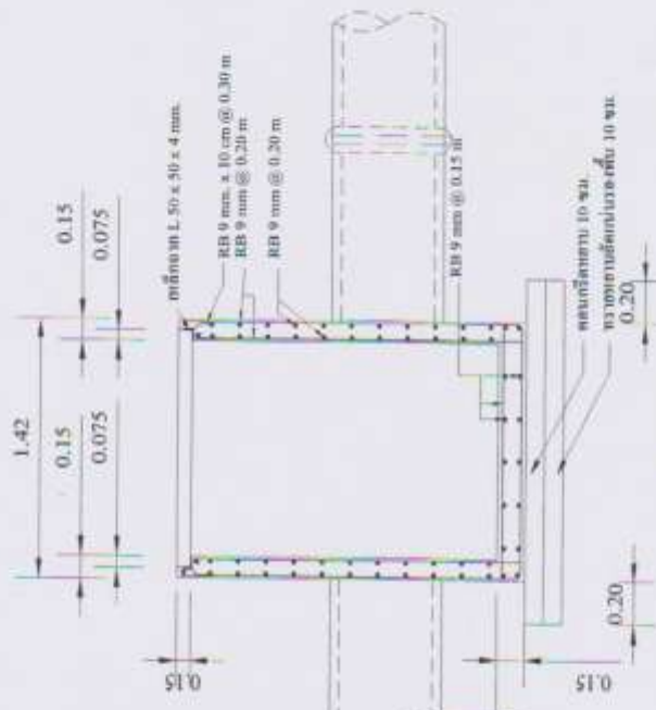
แบบรูปตัด 1-1 ขนาดจริง 1:25
